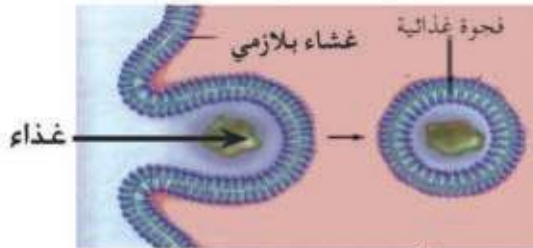
( أ ) ( أ ) الانتهاام او الاكل الخلوي
