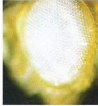
الشكل ( 5 - 21 ) . التغيرات بين لون العين الابيض والاحمر في حشرة ذبابة الفاكهة .
