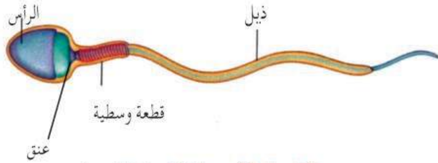
شكل (3-39) . نطفة الانسان الناضجة .
