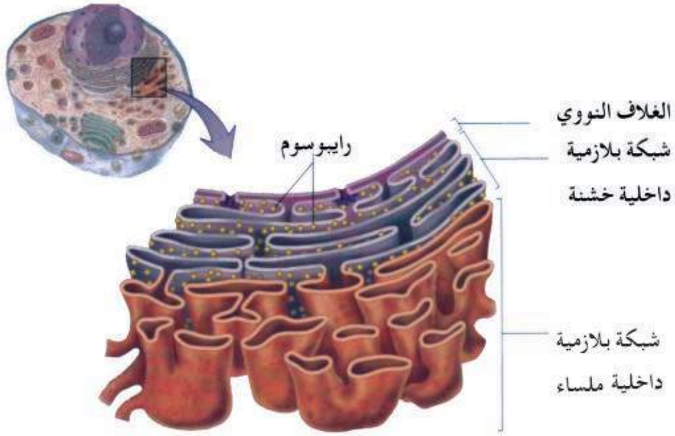
شكل (1-8) الشبكة البلازمية الداخلية الخشنة واللساء وموقعها ضمن الخلية ( للاطلاع ) .
