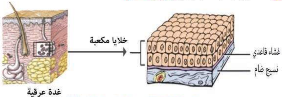
شكل (2-12) النسيج الظهاري المطبق المكعبي .
