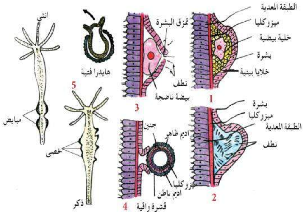
شكل (3-28) . التكاثر الجنسي في الهايدرا 1 - تركيب المبيض . 2 - تركيب الخصية . 3 - الاخصاب . 4 - تكوين جنين . 5 - خروج هايدرا فتية .
