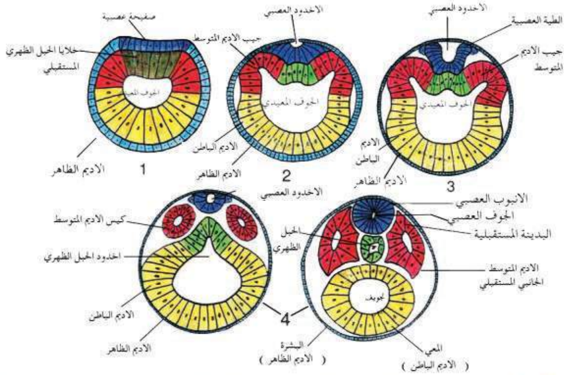
شكل (4-7) . مقاطع مستعرضة في جنين الرميح توضح تكوين الأنبوب العصبي والحبل الظهري والأديم المتوسط والمعى ( للاطلاع ) .
