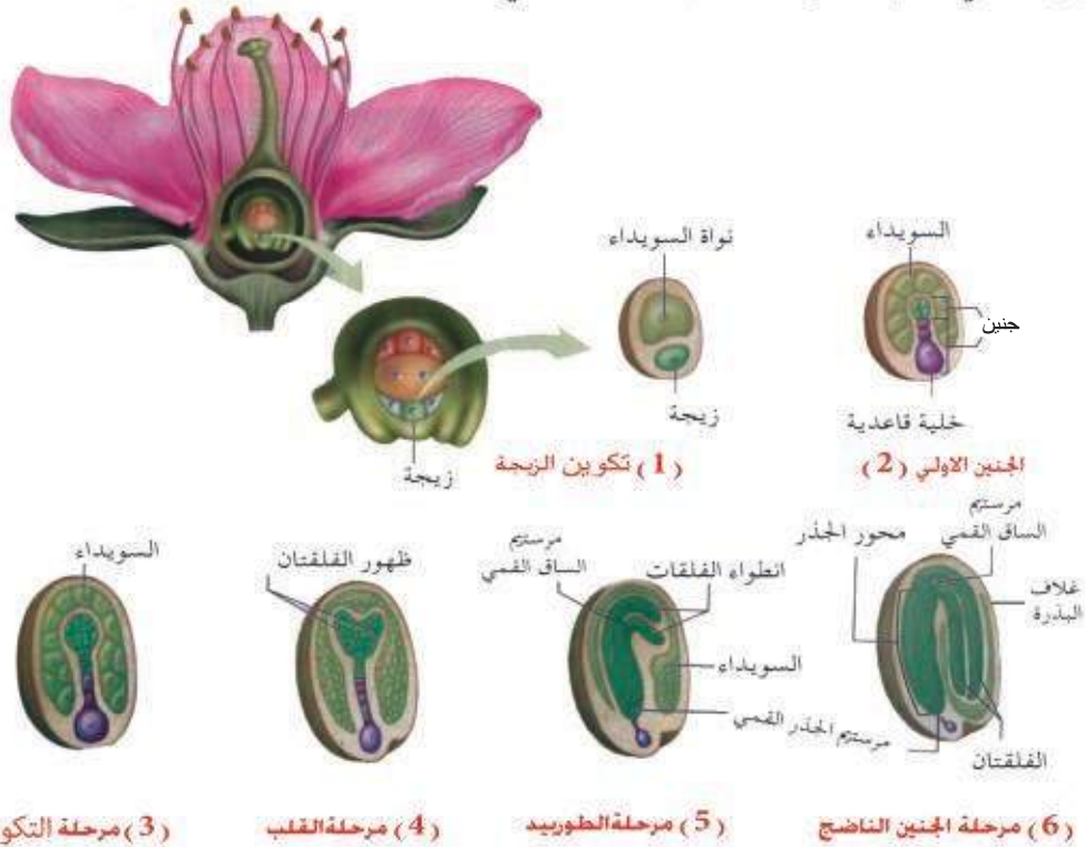
شكل (3 - 18) . التكوين الجنيني لنبات من ذوات الفلقتين .
