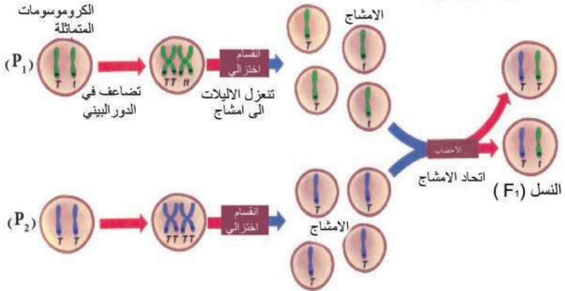
شكل (5-7) يبين انعزال الجين تبعاً لقانون مندل الاول .
