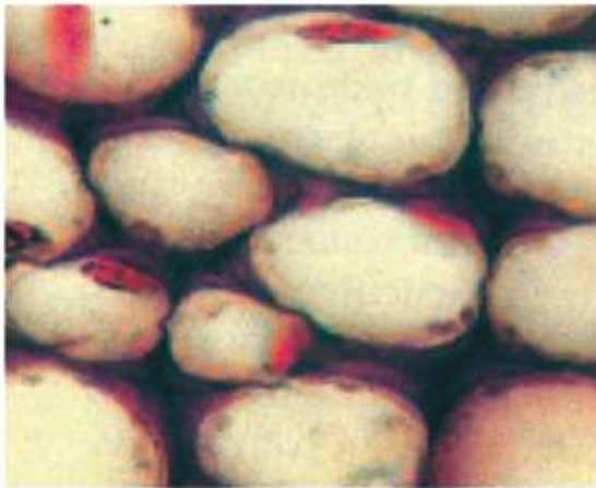
شكل (2-3) . النسيج الكولنكي
