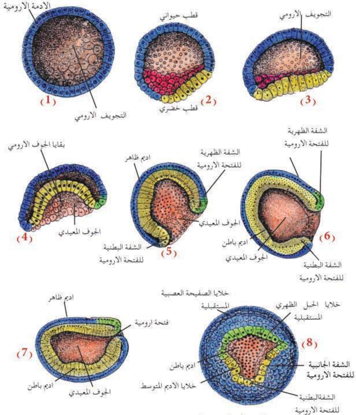
شكل (4-6) . تكوين المعيدة في الريمح ( للاطلاع ) .
