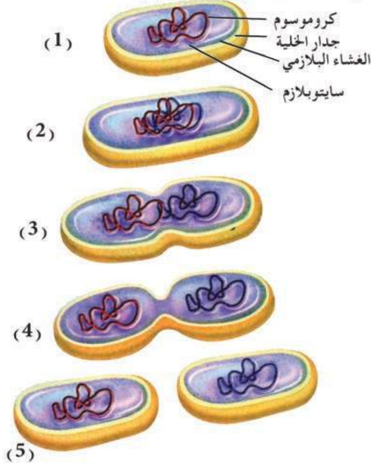
شكل (3-4) . التكاثر اللاجنسي في البكتيريا ( الانشطار الثنائي ) .
