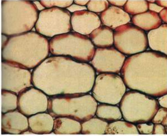
شكل (2-2) . النسيج البرنكي
