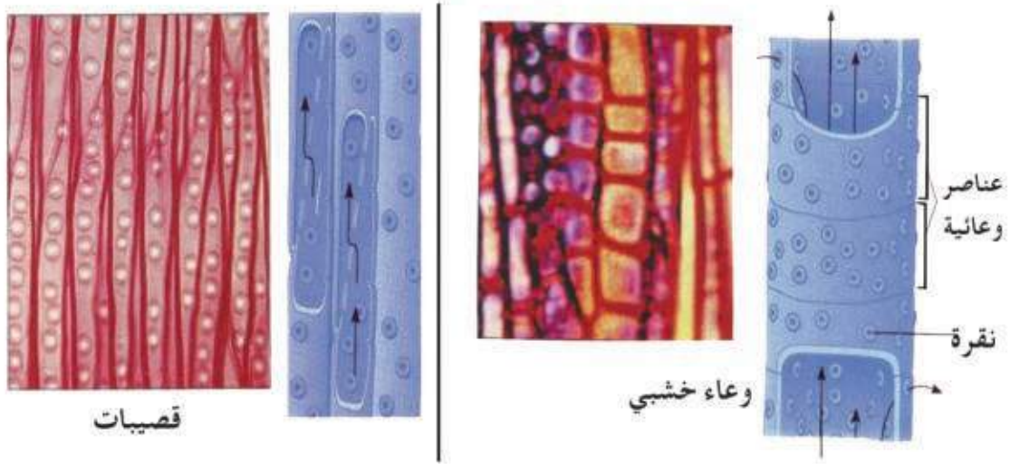
شكل (2-5). القصيبات والاعوية الخشبية ( للاطلاع ) .
