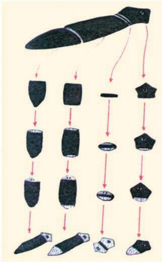
شكل (3-29) . التكاثر اللاجنسي في البلاتاريا ( التقطيع والتجدد ) ( للاطلاع ) .
