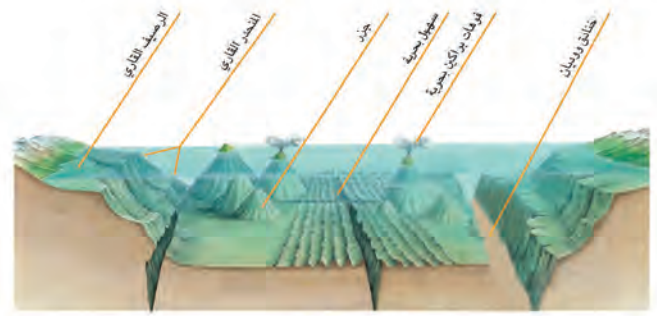
صورة التضاريس لقاع المحيط
